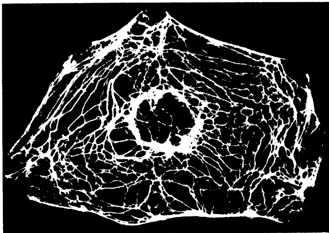
Obr. 50 Fibrilární síť intermediálních filament cyokeratinového typu v sekundární buněčné kultuře ledvinových buněk myšice. Imunofluorescenční mikroskopie
