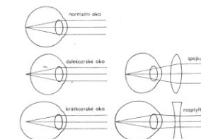
Obr. 219. Schéma dopadu světla do normálního oka a oka s vadou lomivosti. Vpravo korekce pomocí čoček.
