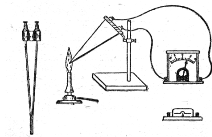
Obr.5.17 a) Termočlánek.
