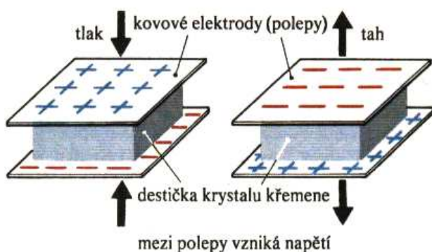
Obr.4.46. Piezelektrický jev.
