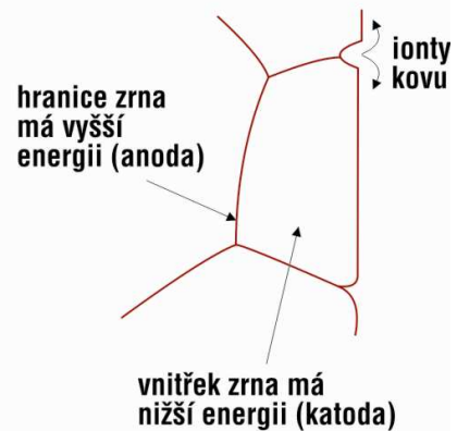
Obr.1.9. Korozní dvojice hranice zrna – vnitřek zrna
