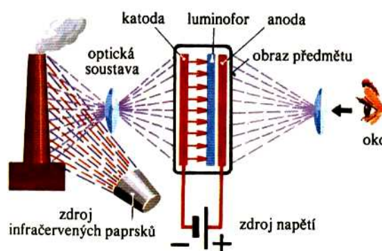
Obr.4.53. Přeměna infračerveného záření na viditelné světlo.
