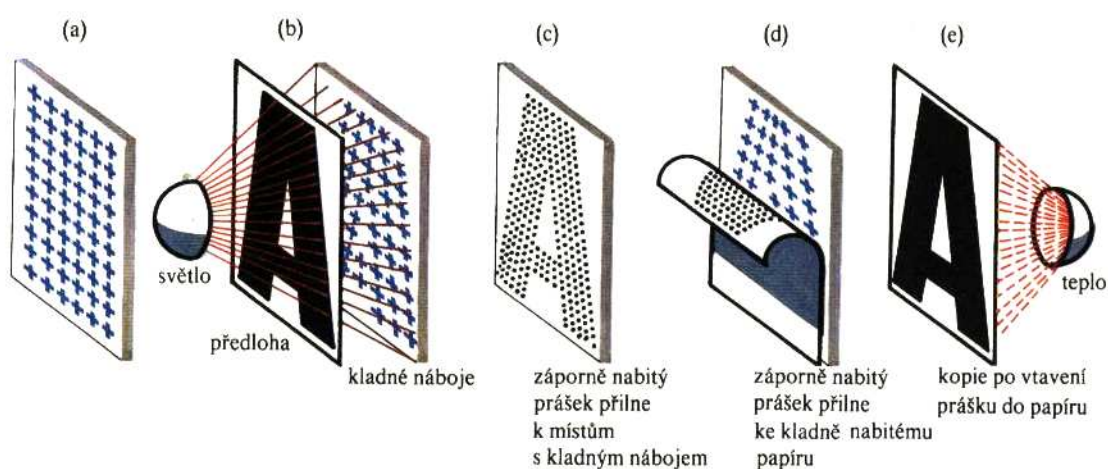
Obr.4.1. Princip činnosti xerografie.
