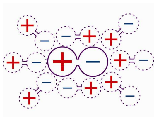
Obr.1.1a) Vznik klastru
