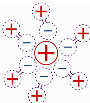
Obr.1.1.b) Disociovaný iont
