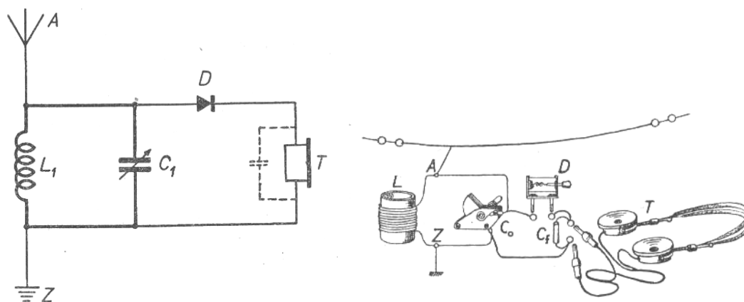
Obr.5.49. Schéma krystalového přijímače.
