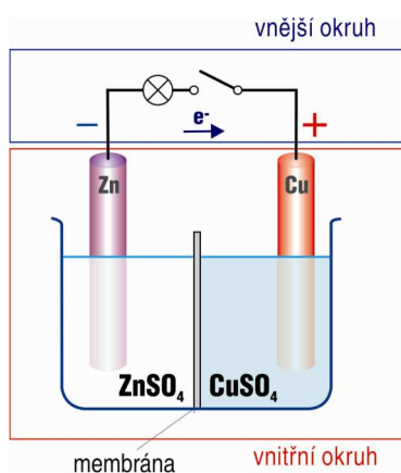
Obr.1.7a) Danielův článek
