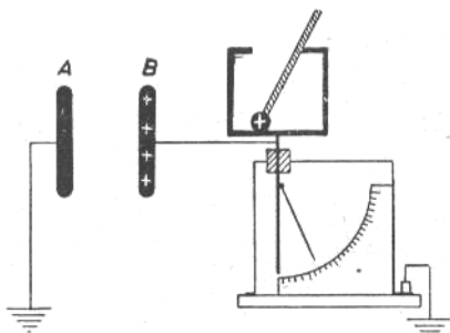
Obr. 5.12. Vlastnosti elektrického kondenzátoru.
