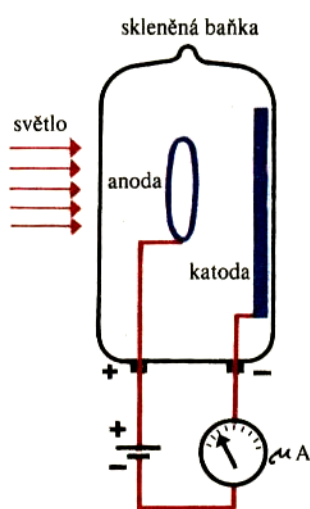
Obr.4.50. Schéma fotonky.
