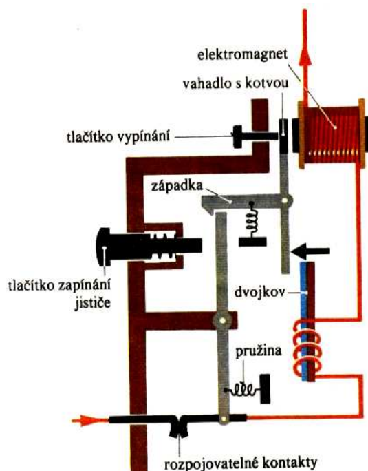
Obr.4.30. Jistič.
