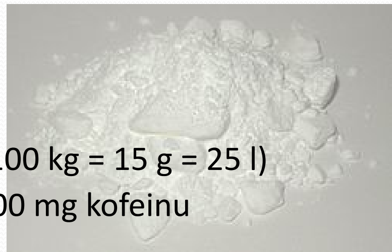
Obr. 6. Bezvodý Kofein
