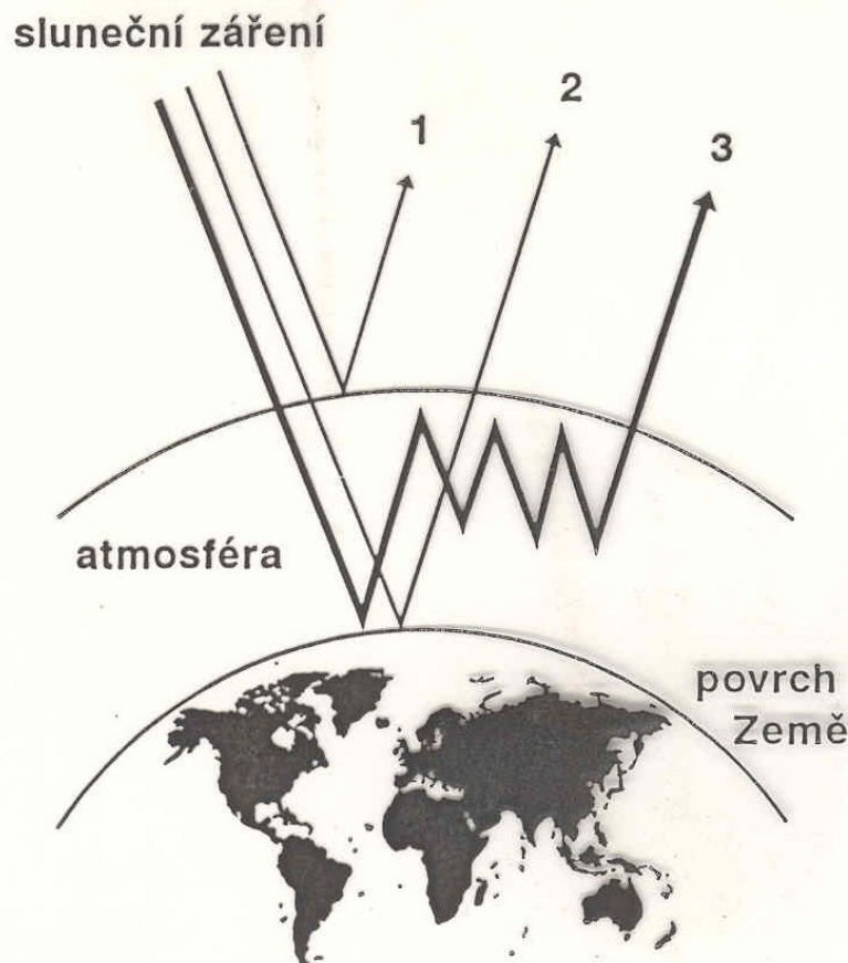
Obr. 24. Skleníkový jev
