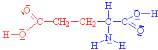
kyselina glutamová
