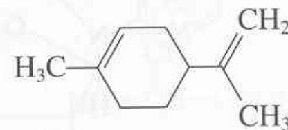
limonen
