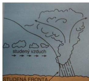
Obrázek 2 Vertikální řez studenou frontou (ilustrace)
