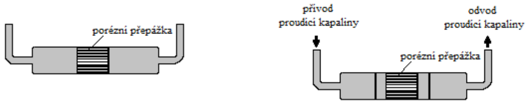
Obr. 7.17: Schéma uspořádání při měření potenciálu proudění:
