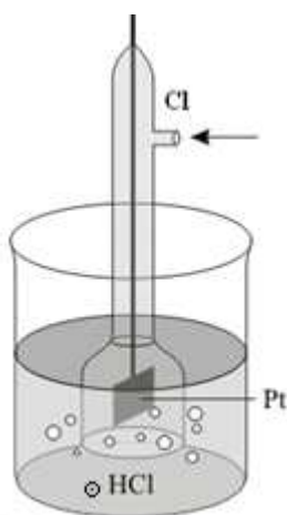
Obr. 6. 18: Příklad aniontové elektrody 1. druhu
