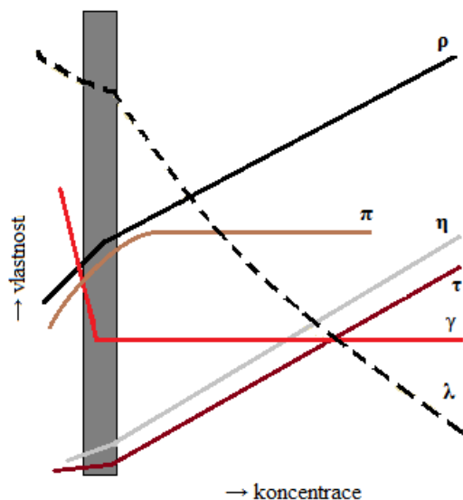
Obr. 7.5: Koncentrační závislost vybraných fyzikálních vlastností vodného roztoku dodecylsulfátu sodného.
