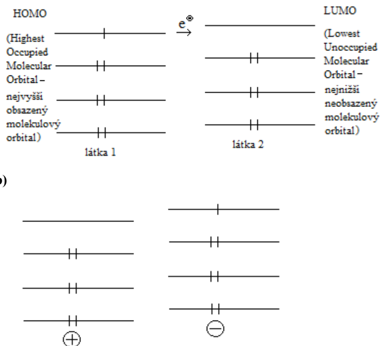
Obr. 8.12: Přeskok e^- mezi dvěma látkami.
