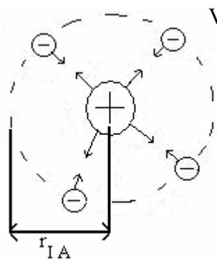
Obr. 6. 7: Aproximace reálné situace působením iontové atmosféry.
