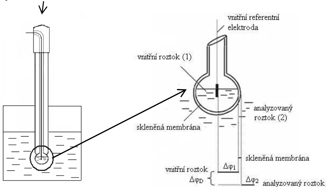
Obr. 6. 23: Skleněná elektroda.
