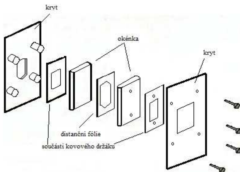
Obr. 8.11: Rozebíratelná kyveta pro měření vibračně-rotačních spekter kapalin. Převzato z [16].
