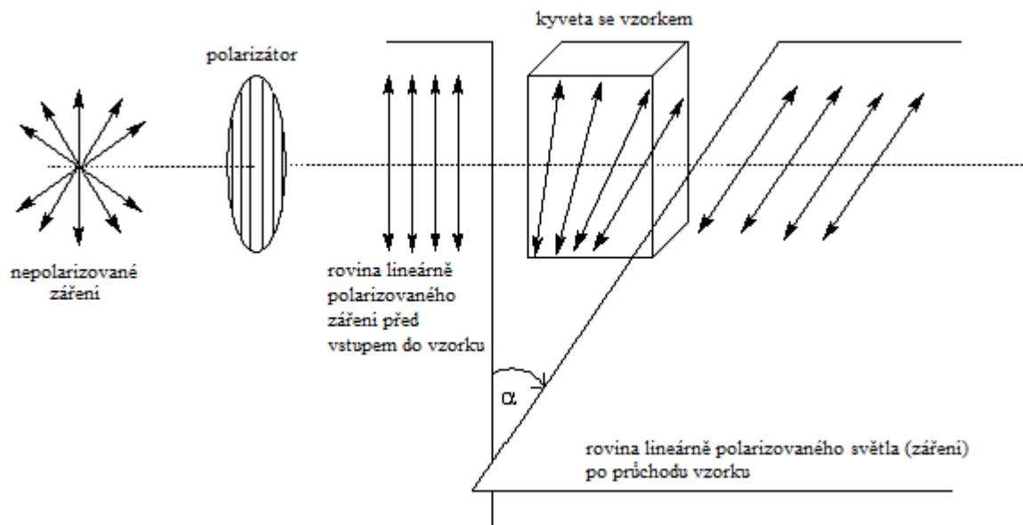
Obr. 8.4: Chování záření při průchodu opticky aktivním vzorkem. α ...optická otáčivost
