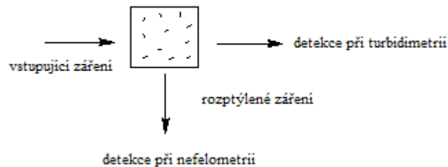
Obr. 8.19: Chování záření při průchodu jemnou suspenzí nebo koloidním roztokem.
