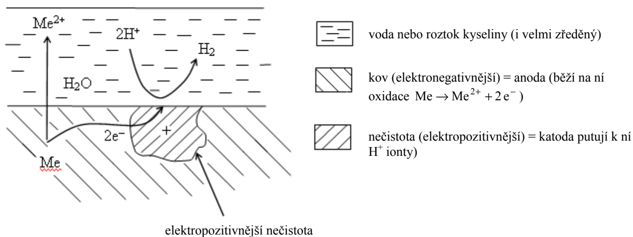
Obr. 6. 45: Elektrochemická koroze.
