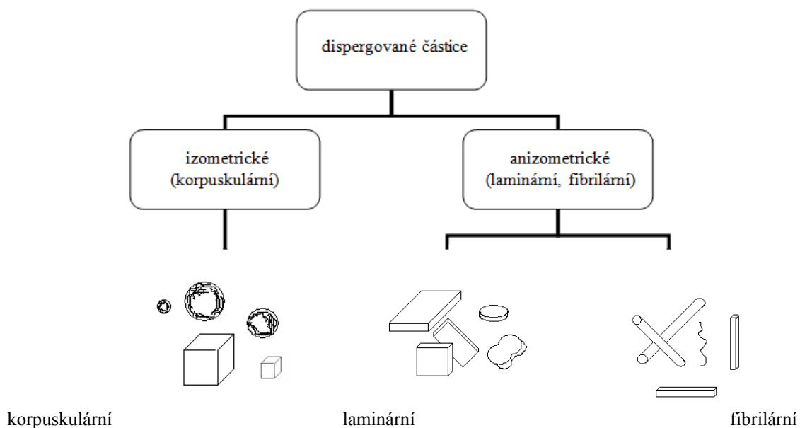
Obr. 7.2: Typy dispergovaných částic podle tvaru.
