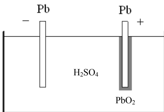
Obr. 6. 50: Nabítý olověný akumulátor – katoda je čisté olovo, anoda je pokryta \text{PbO}_2 [66].
