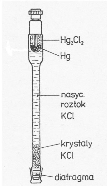
Obr. 6. 19: Kalomelová elektroda [93].
