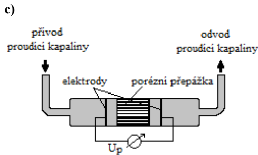
Obr. 7.17: Schéma uspořádání při měření potenciálu proudění:
