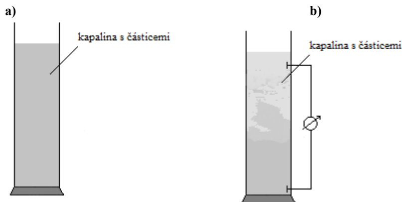
Obr. 7.18: Schéma uspořádání při měření sedimentačního potenciálu
