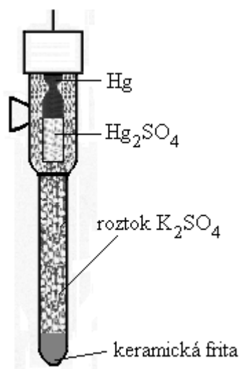
Obr. 6. 21: Merkursulfátová elektroda.
