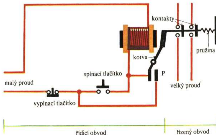
Obr.4.8. Elektromagnetický stykač.
