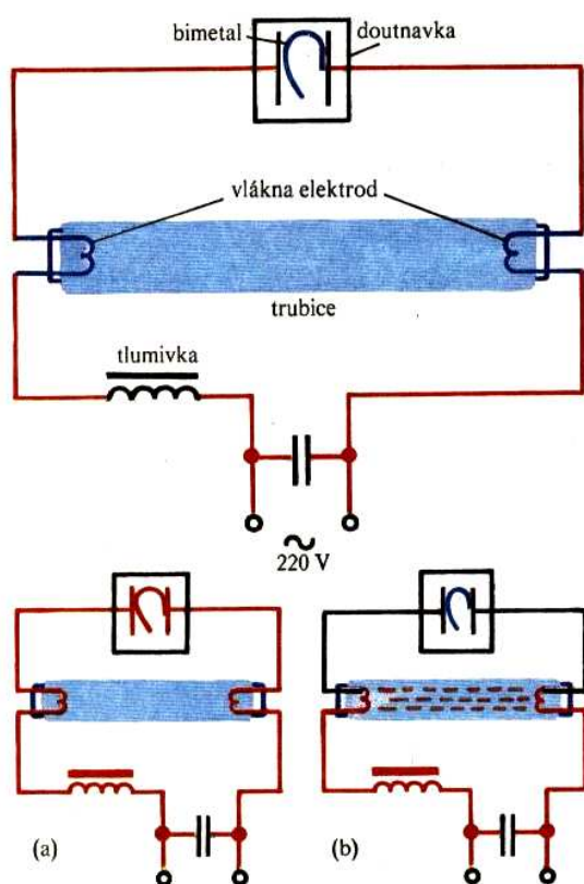
Obr.4.45. Zářivka
