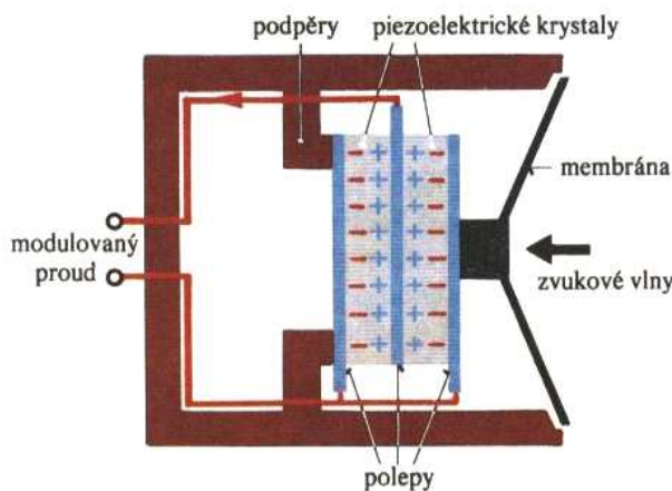
Obr.4.59. Piezoelektrický mikrofon
