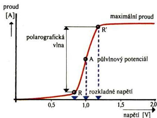
Obr.4.27. Polarografická křivka
