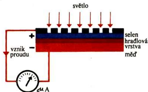
Obr.4.48. Hradlový článek.
