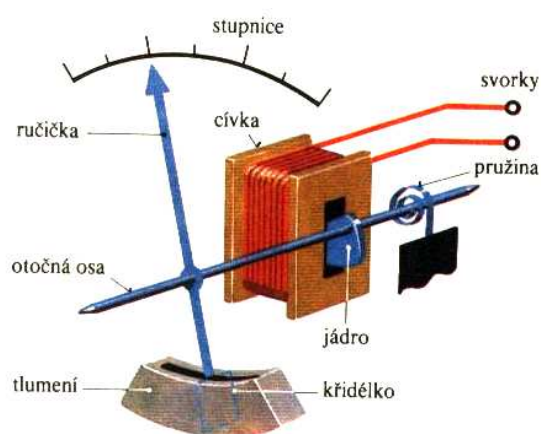
Obr.4.20. Elektromagnetický měřicí přístroj.
