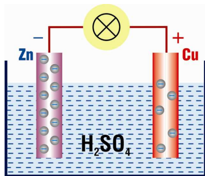
Obr.1.5a) Voltův článek
