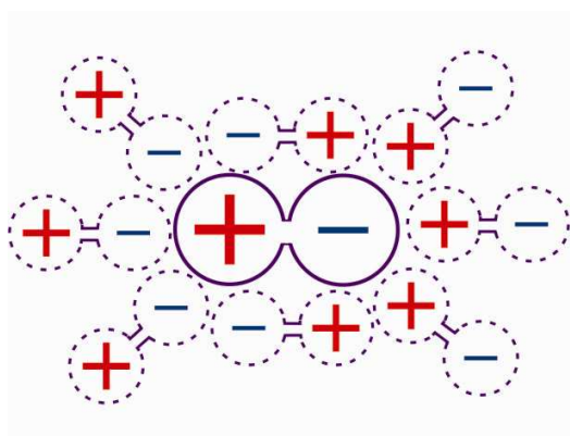
Obr.1.1a) Vznik klastru
