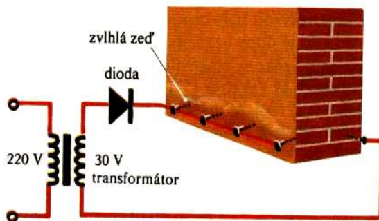
Obr.4.25. Vysoušení zdi pomocí elektrolýzy.
