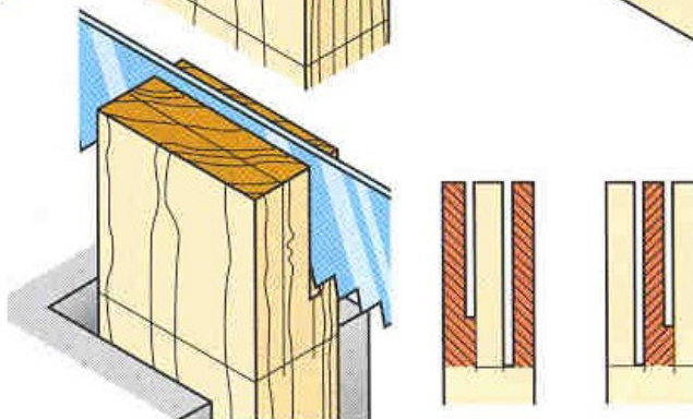
řezání čepu rozporu
