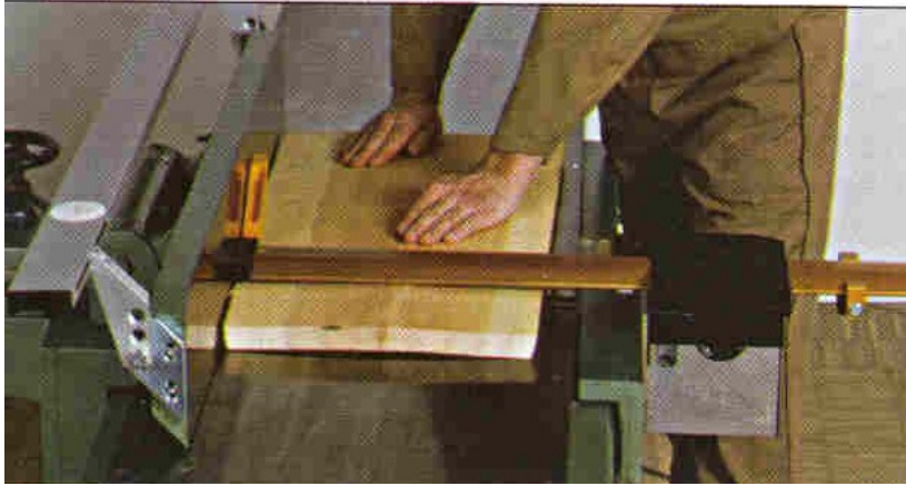
Hoblování dřeva
