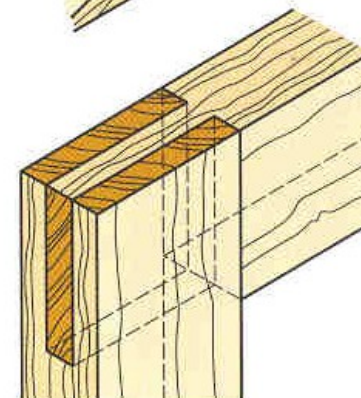
slepení a očištění spoje
