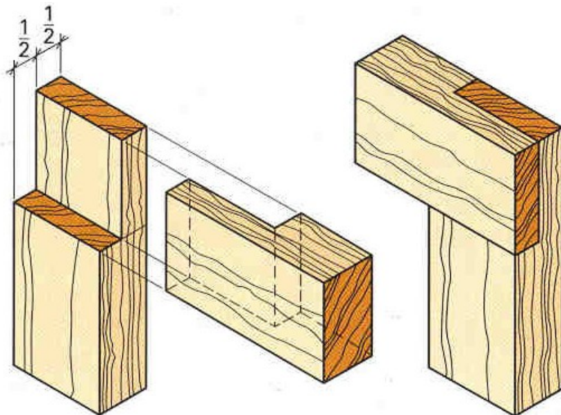
Přeplátování
