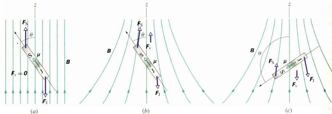
Obr. 41.9 Magnetický dipól, znázorněný jako tyčový magnet se dvěma póly (a) v homogenním magnetickém poli a (b, c) v poli s gradientem v z-ovské směři.
