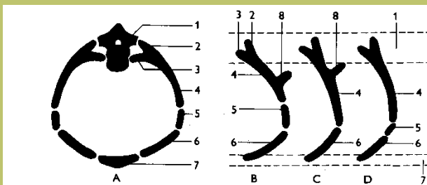
Obr. 23: Schéma organizace žebere amniotů. A - hrudní segment v předozadní projekci, B - třídlínné žebro plazů, C - dvoudílné žebro ptáků, D - třídlínné žebro ptakopyška a mravenečnicka. 1 - topografická poloha obratle, 2 - tuberculum costae, 3 - caput costae, 4 - vertebrocostale, 5 - intercostale, 6 - sternocostale, 7 - topografická poloha sternu, 8 - processus uncinatus. Upraveno podle Portmann, 1965.
