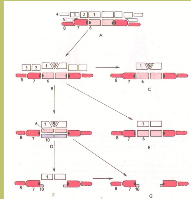
Obr. 37: Schéma evoluce lopatkového pásmo. Šipky naznačují předpokládaný směr vývoje. A - ryby, B - primitivní obojživelníci, C - žáby, D - plazi a vejcorodí savci, E - moderní plazi a ptáci, F - zivorodí savci, G - specializovaní savci. 1 - clavicula, 2 - cleithrum, 3 - supracleithrum, 4 - posttemporale, 5 - postcleithrum, 6 - procoracoid, 7 - scapula, 8 - suprascapula, 9 - interclavicula, 10 - metacoracoid (processus coracoideus), černě je vyznačena kloubní jamka pro humerus. Upraveno podle Remaneho et al., 1972.
