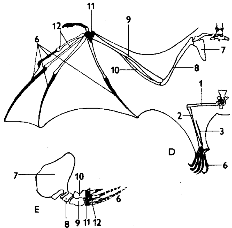
Obr. 175: Stavba kostry končetin u různých savců. A - zadní končetina plaskochodce (opice), B - zadní končetina prstochodce (pes), C - zadní končetina kopytníka (kůň), D - kostra končetin u letounů (kaloň), E - kostra přední končetiny delfína ( Tursiops ). 1 - femur, 2 - tibia, 3 - fibula, 4 - tarsalia, 5 - metatarsalia, 6 - phalanges, 7 - scapula, 8 - humerus, 9 - radius, 10 - ulna, 11 - carpalia, 12 - metacarpalia. Upraveno podle Ziswillera, 1976.
