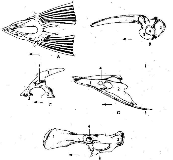
Obr. 38: Nástin evoluce pánevního pásmo obratlovců. A - kapr shora, B - skokan zleva, C - varan zleva, D - hotub zleva, E - králík zleva. Šipky vyznačují směr k hlavě. 1 - os ilium, 2 - os ischiū, 3 - os pubis, 4 - acetabulum (kloubní jamka pro femur). C.) podle Ihleho et al., 1971, ostatní jsou originály.
