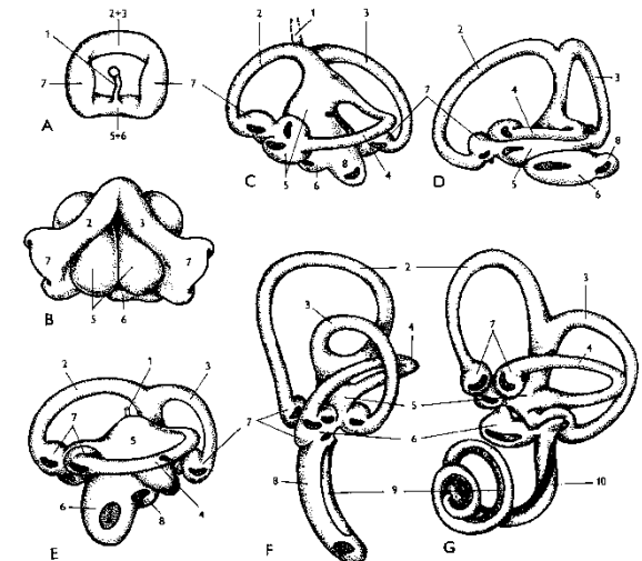
Obr. 34 Blanitý labyrint vnitřního ucha. A – sliznatky (Mysxinoidea), B – mihule (Petromyzontida), C – pa- ryby (Chondrichthyes), D – paprskoploutvé ryby (Actinopterygii), E – bezocasí obojživelníci (Anura), F – ptáci (Aves), G – savci (Mammalia). 1 – ductus endolymphaticus, 2 – přechod, 3 – zadní a 4 – po- stranní polokružná chodba, 5 – utriculus, 6 – sacculus, 7 – ampule polokružných chodeb, 8 – lagena, 9 – papilla basilaris, resp. Cortiho orgán, 10 – hlemýžď (cochlea). Oblasti se smyslovými buňkami (ma- culae) jsou ohraničeny a vytečkovány.
