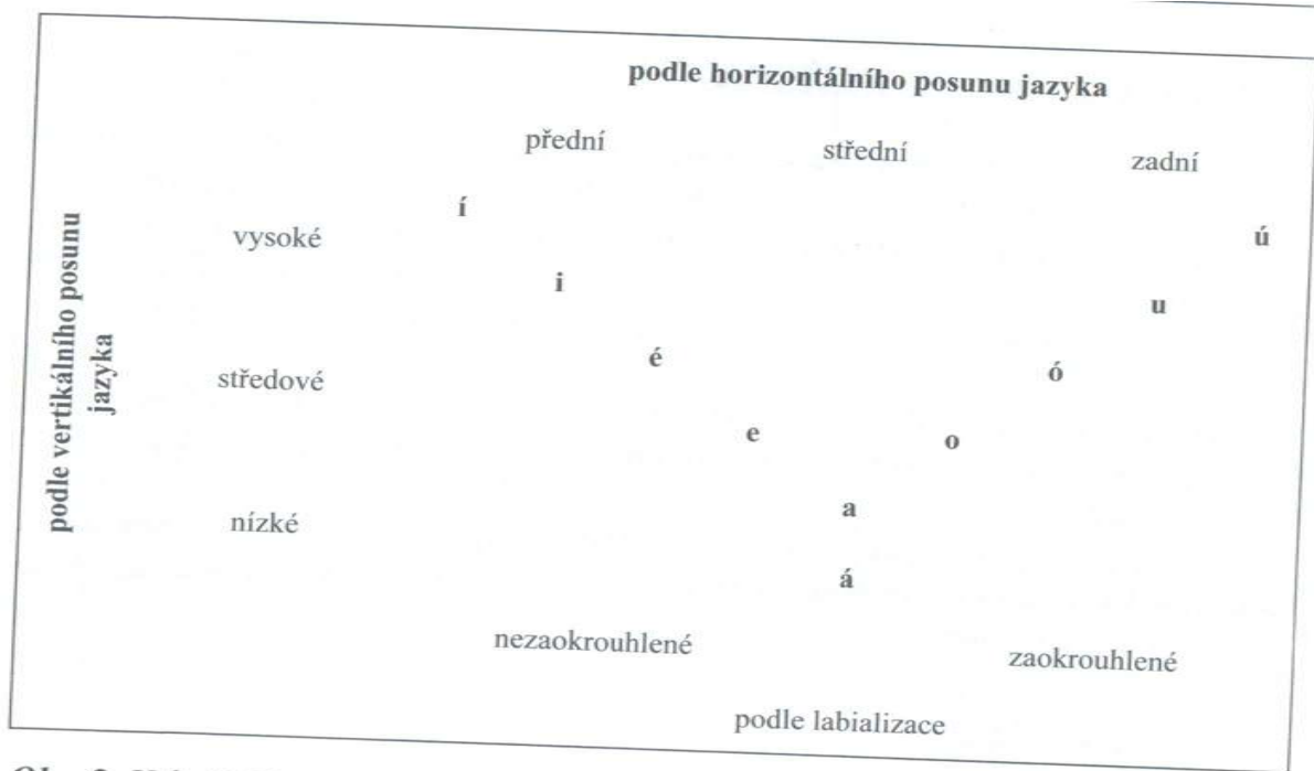
Obr. 2 Vokalický trojúhelník
