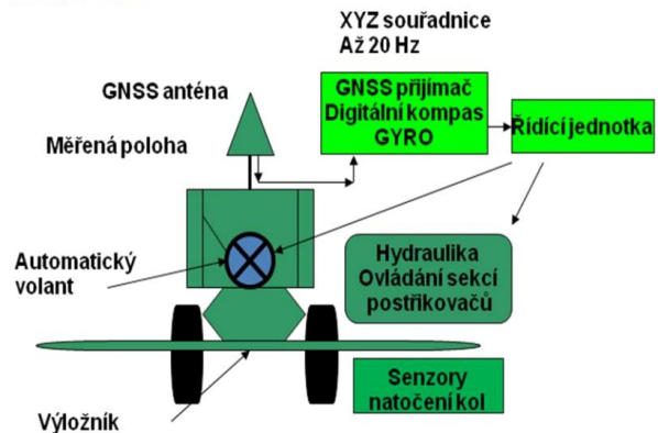
Obr. 11: Buldozer s nainstalovaným řídicím systémem s GPS (vlevo). Využití GNSS v přesném zemědělství – pohyb zemědělského stroje (vpravo). Zdroj: http://www.crr.vutbr.cz/system/files/brozura_08_1009.pdf
