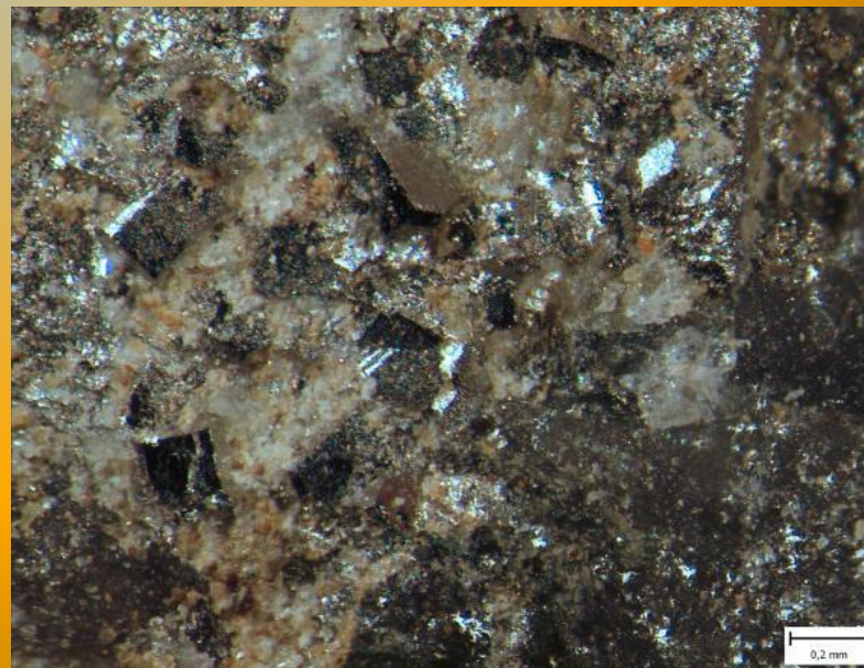
Rombické krystaly arzenopyritu - Mokrsko
