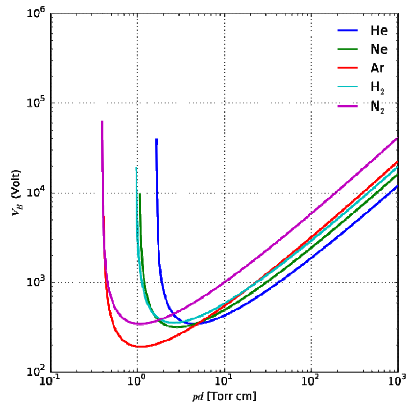
Paschenova křivka pro různé plyny (1 torr = 133,3 Pa)
