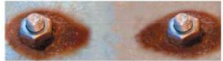
Obr. 1 Příklad bimetalické koroze šroubů z korozivzdorné oceli použitých pro spojení žárově zinkovaných dílů
