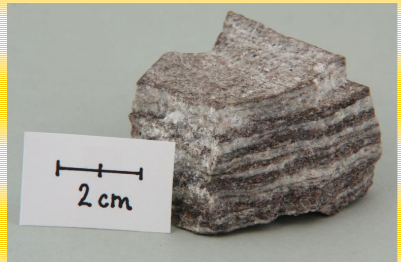
Páskovaný granulit, tmavé pásy s obsahem biotitu, Horní Bory.
