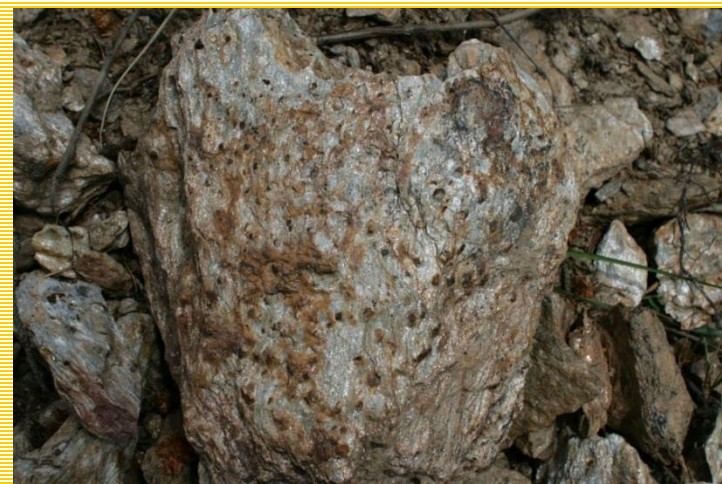
Porfyroblasty granátu ve svoru s výraznou foliací, Sobotín.
