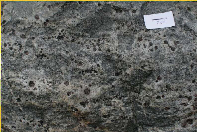
Migmatitizovaná tula s porfiroblasty granátu, Tábor.
