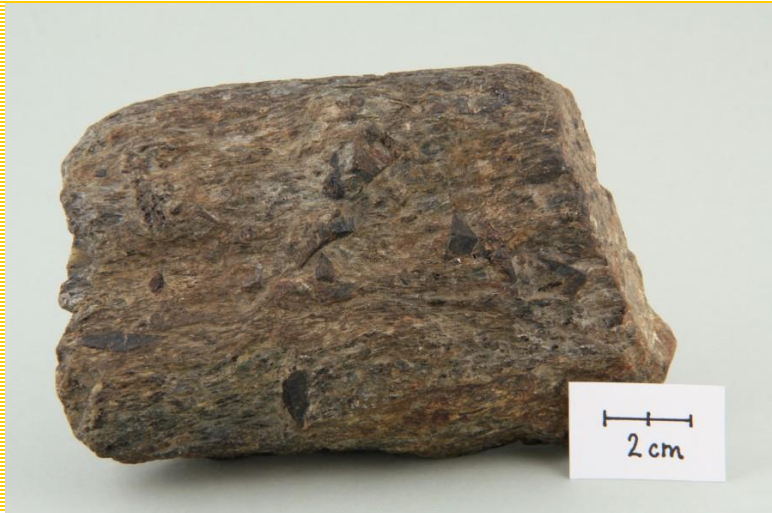
Staurolitový svor, Vranov.
