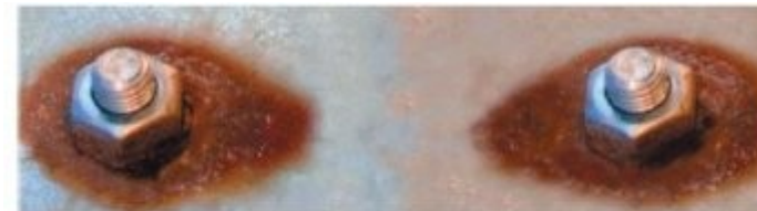
Obr. 1 Příklad bimetalické koroze šroubů z korozivzdorné oceli použitých pro spojení žárově zinkovaných dílů
