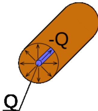
Válcový kondenzátor
