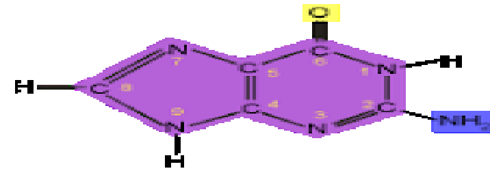
Guanin (G)
