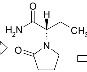
levetiracetam
