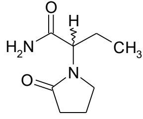
etiracetam
