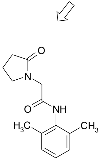
nefiracetam
