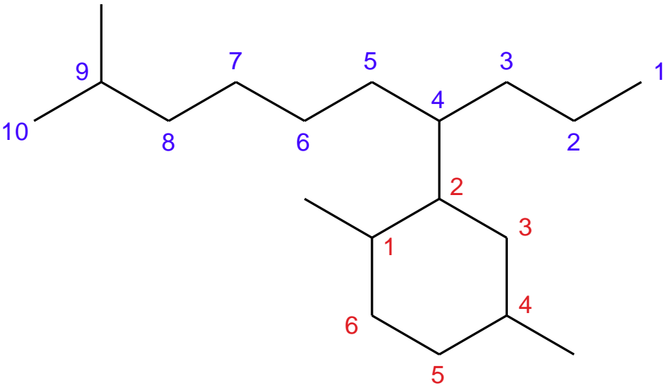
1,4 -dimethyl- 2 -( 9 -methyldekan- 4 -yl)cyklohexan
