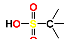
sulfová kyselina
