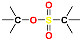
sulfonát ester
