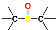
sulfoxid
