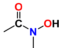
hydroxamová kyselina
