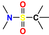
sulfonamid (1°,2°,3°)
