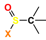
sulfinylhalogenid
