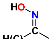
oxim
