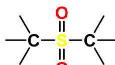
sulfon
