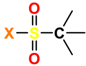
sulfonylhalogenid
