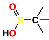
sulfinová kyselina
