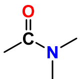
amid (1°,2°,3°)
