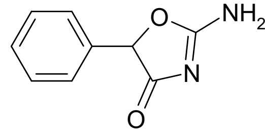
2-amino-5-fenyl-1,3-oxazol-4(5H)-on
