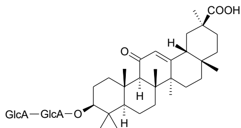
glycyrrhizová kyselina
