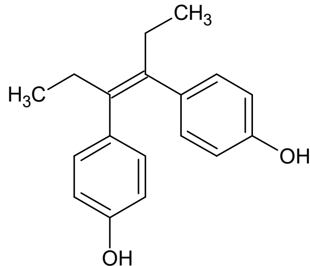
cis -diethylstilbestrol
