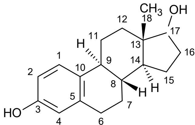
estradiol
