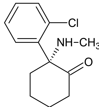
2-(2-chlorophenyl)-2-(methylamino)cyclohexanone
