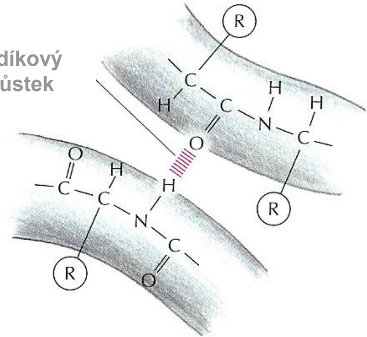
van der Waalsova síla
