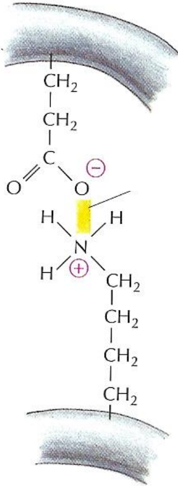
iontová vazba
