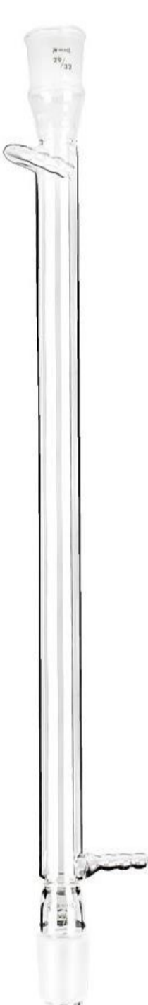
CHLADIČ LIEBLINGŮV
