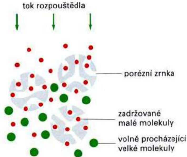
(B) GELOVÁ CHROMATOGRFIE
