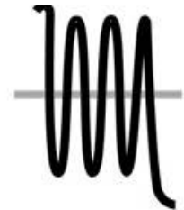
Chemokinové receptory
