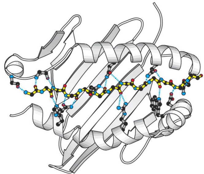
MHC II
