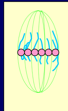
mitotická metafáze
