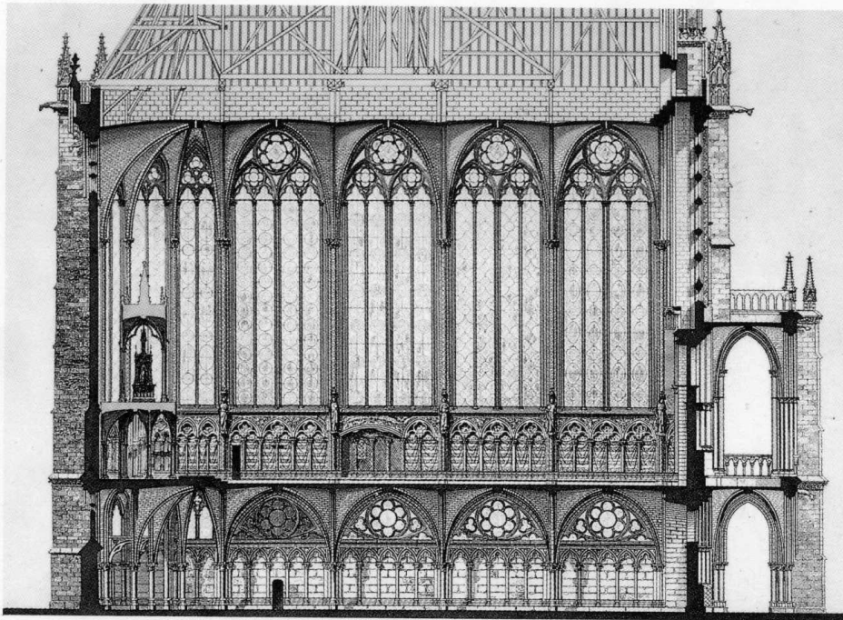
408 – Paris, Sainte-Chapelle – Längsschnitt
