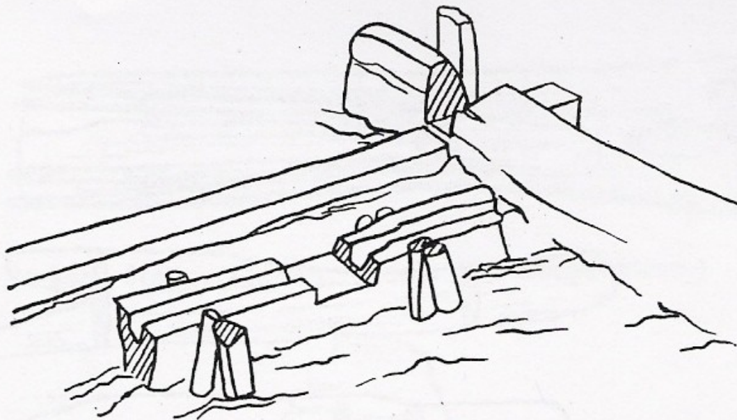
Lamka — trdlice z Gdańska, pol. 11. stol. (Podle J. Kamińskiej a A. Nahlika.)
