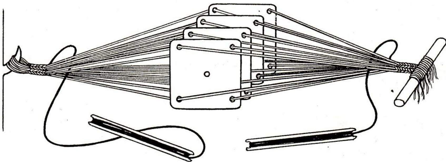
Schéma výroby pasů na karetkách.
