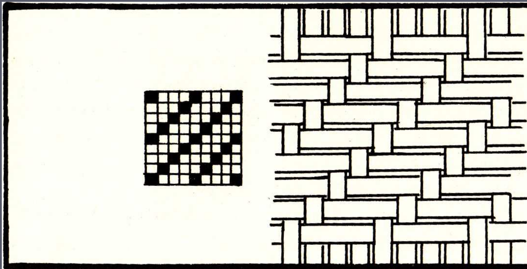
Schéma tkaniny ve vazbě čtyřvazného útkového kepru
