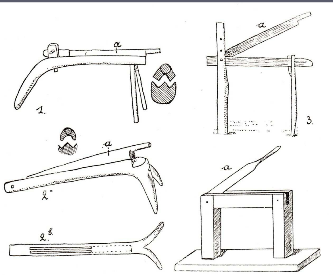
264. Międlice. 1. Gornja Batina pow. Złatar, Chorwacja północna. Muz. etn. w Zagrzebiu. 2. Gnieździłowo pow. Głębokie, Białoruś. 3. Kumarica i Kuriło, NE od Sofii, Bułgaria. 4. Ust'-Nicyńskoje obw. tiumeński, Syberia zachodnia. 1—3. rys. autor; 4. „Żiwaja Starina”, t. 4, 1894, s. 57, fig. 1.
