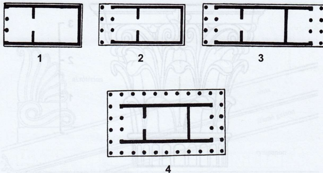
5. Typy řeckých chrámů podle půdorysu. 1 chrám in antis, 2 prostylos, 3 amfiprostylos, 4 peripteros.
