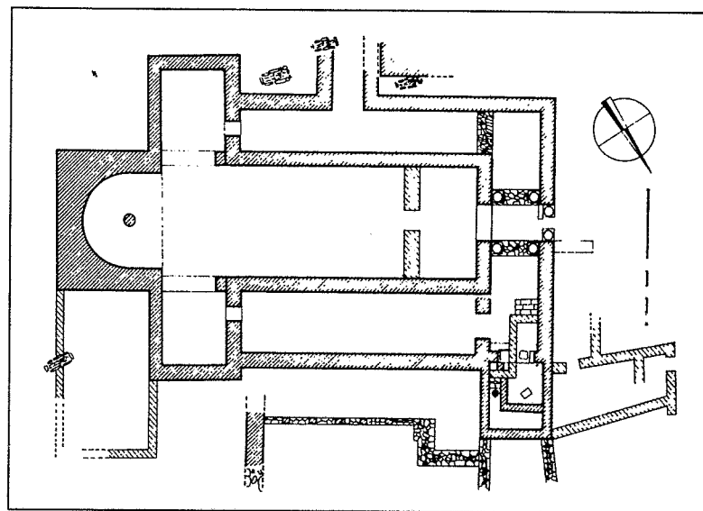
Plán baziliky v Reccopolis
