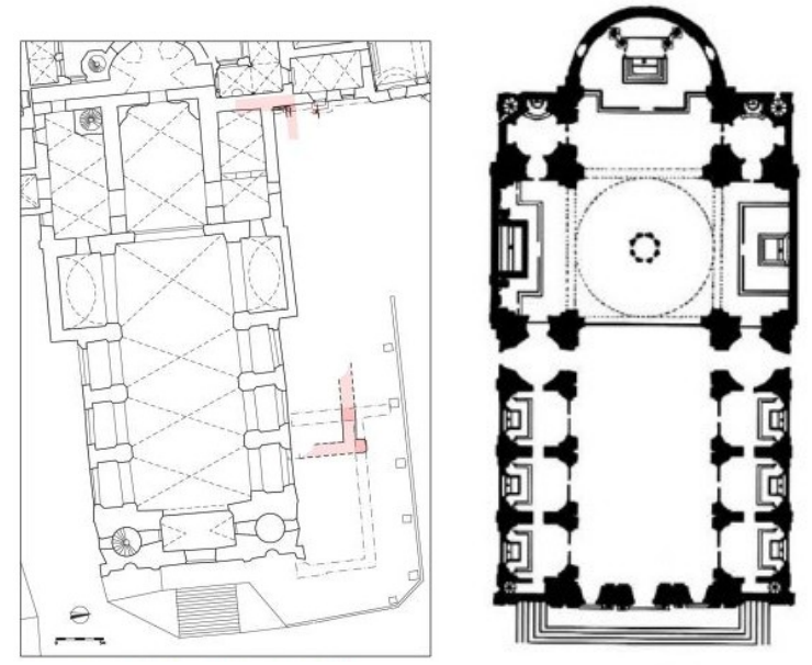
Dominikánský kostel sv. Michala: v Brně nejbližší jezuitským vzorům – Il Gesù (půdorys) a Vídeň
