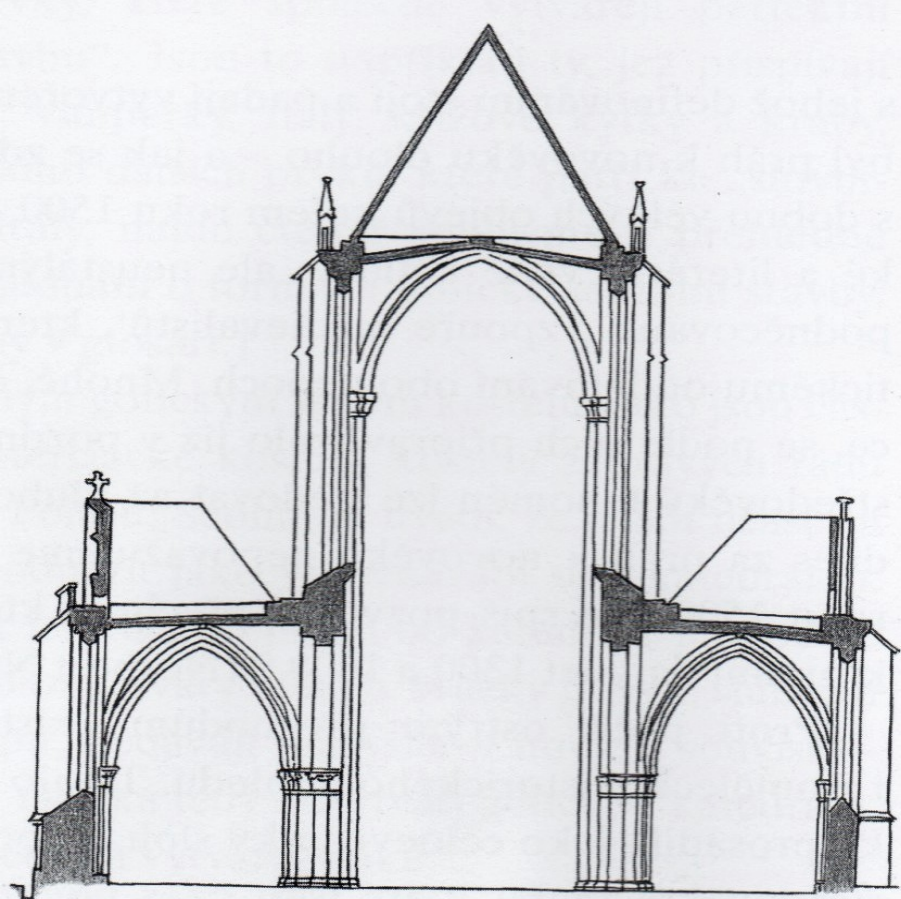
bazilika bez opěrného systému příčný řez (Magdeburk)
