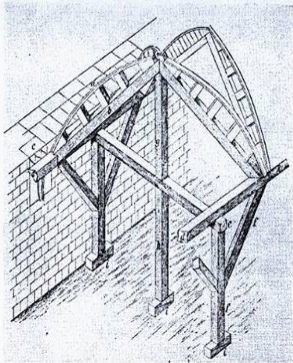
Ramenátová konstrukce pro sestrojování gotické žebrové klenby podle: G. Ungewitter, K. Mohrmann, Lehrbuch der gotischen Konstruktionen, I, Leipzig 1890, str. 118.
