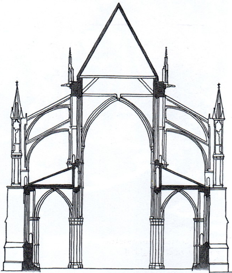
bazilika s opěrným systémem příčný řez (Remeš)
