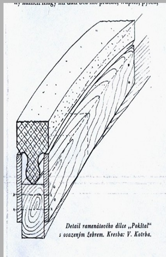
Rekonstrukce původní ramenátové konstrukce pro sestrojování gotické žebrové klenby — „Pokštal“, „truhlíkový ramenát“. Kresba: V. Kotrba
