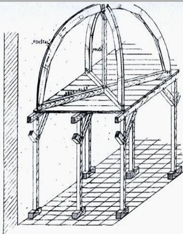
Rekonstrukce původní ramenátové konstrukce pro sestrojování gotické žebrové klenby — „Pokštal“, „truhlíkový ramenát“. Kresba: V. Kotrba
