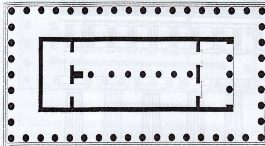
II. 21. Héřin Chrám I v Paestu (tzv. basilika), po polovině 6. stol. př. Kr.
