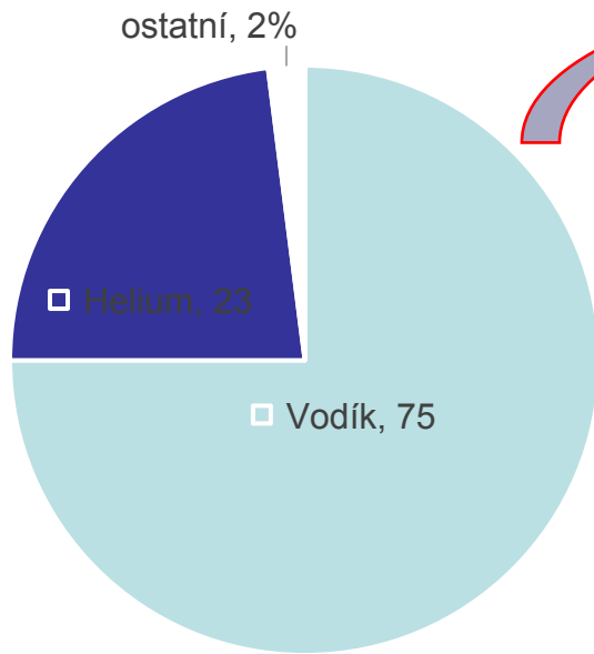
Složení vesmíru
