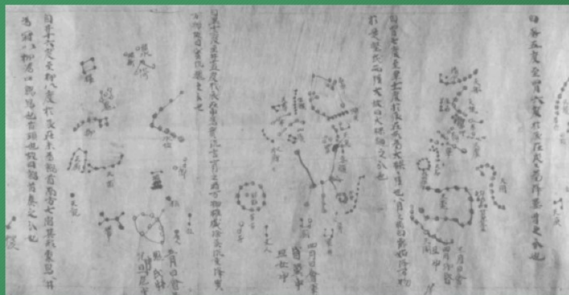
hvězdná mapa
