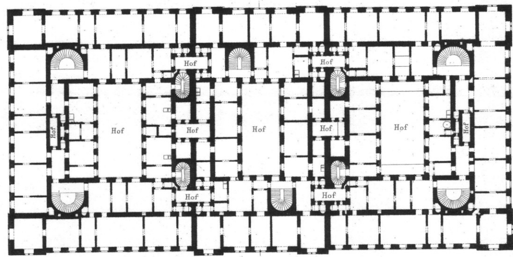
Grundriss des I. Stockes.
