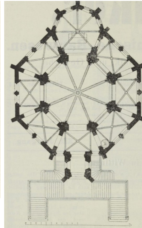
Fig. 2. Grundriss vom Hochparterre.
