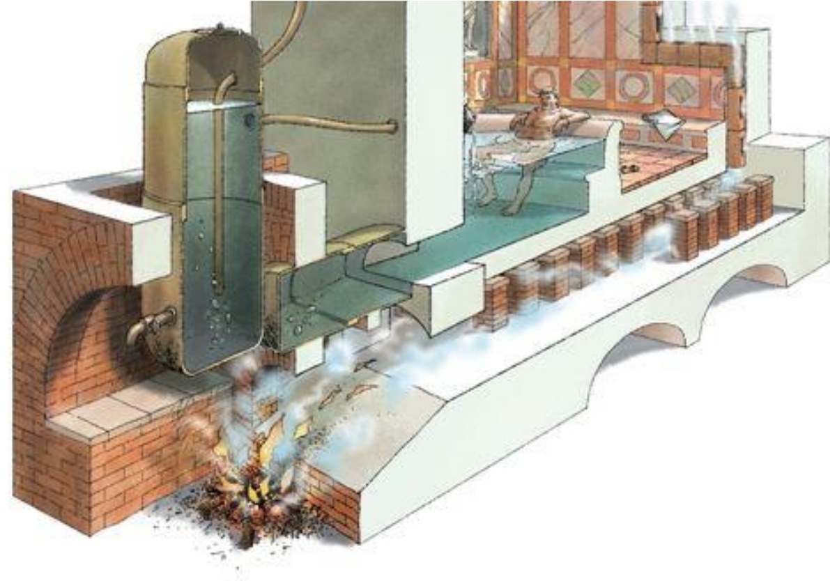
Hypokaustum, rekonstrukce
