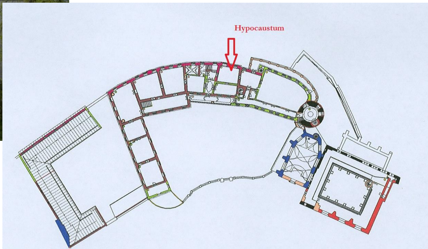
Olomouc, býv. Kapitulní děkanství, půdorys 1. patra
