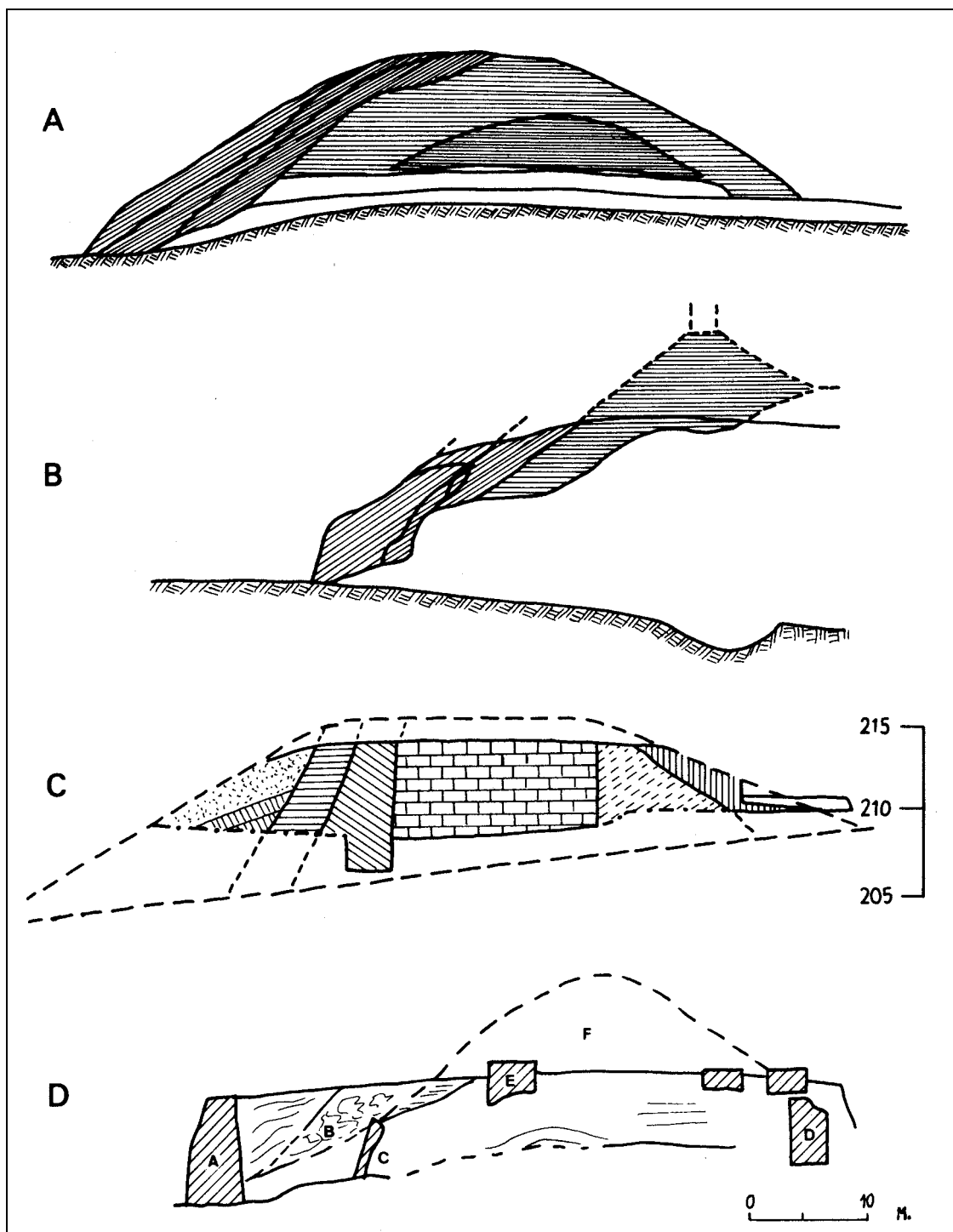
Profily fortifikačních náspů střední doby bronzové
