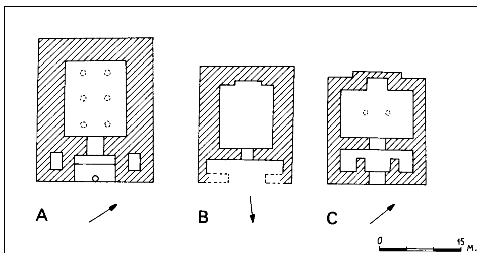
Srovnání chrámových půdorysů střední doby bronzové
