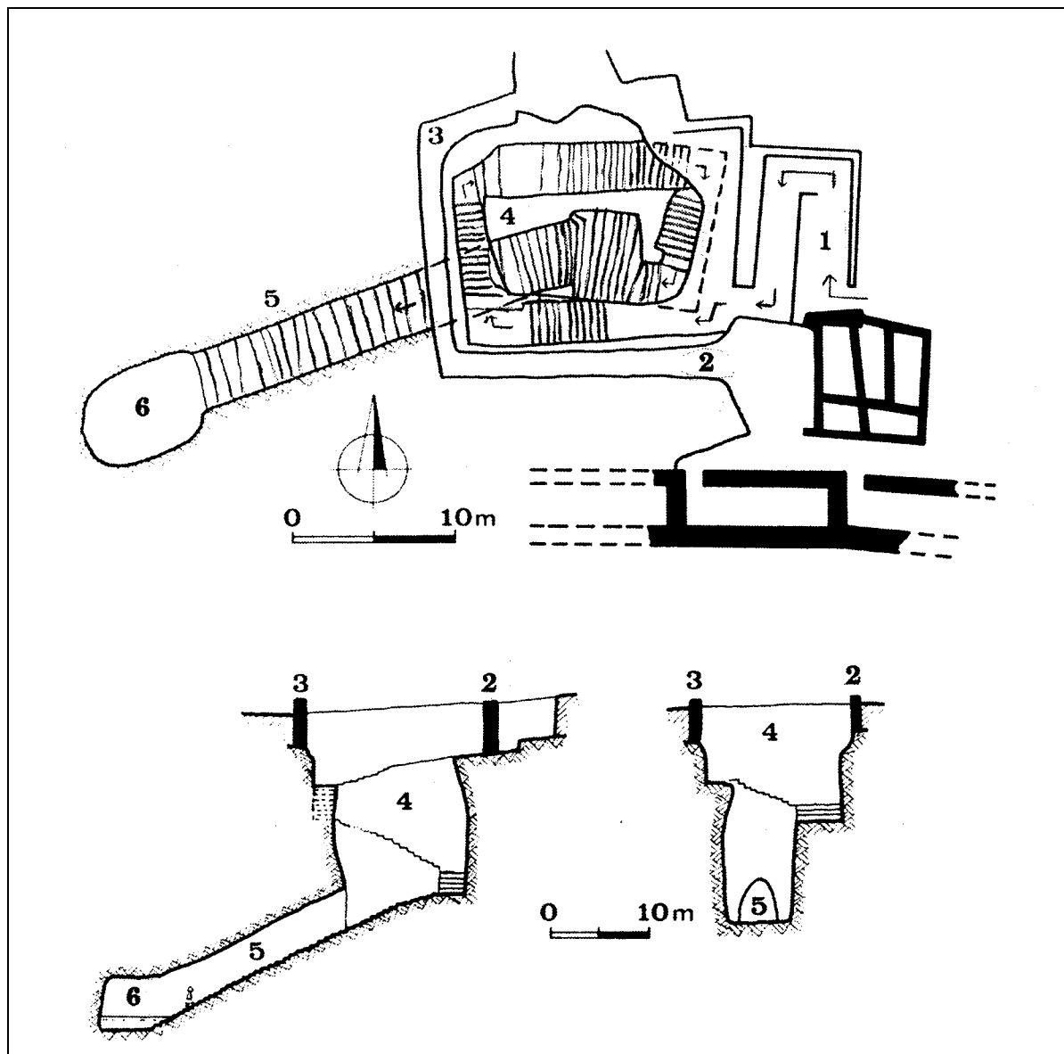
Chasór. Plán vodovodního systému
