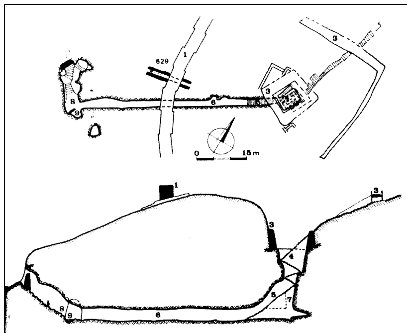
Megido. Plán vodovodního systému (vrstva IVA)
