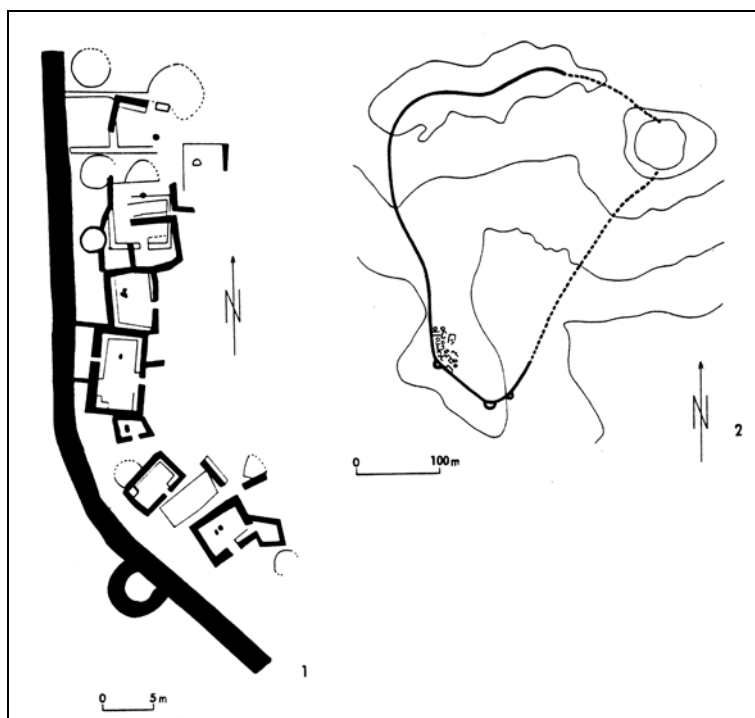
Arad. Městské opevnění
