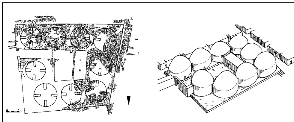
Obilnice v Bét Jerach
