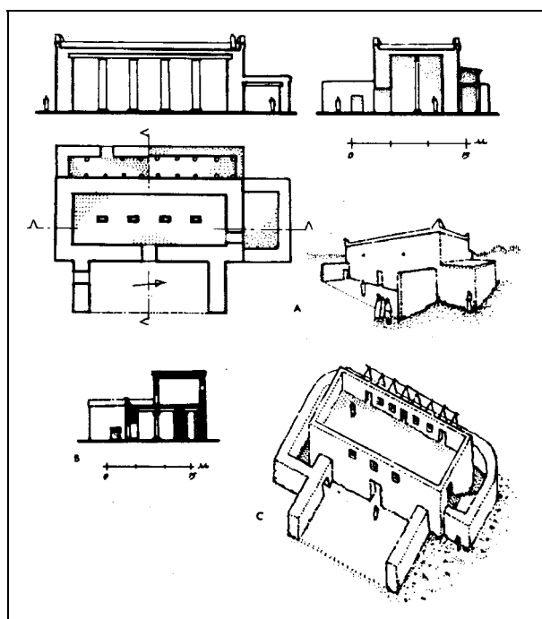
Aj. Chrám na akropoli
