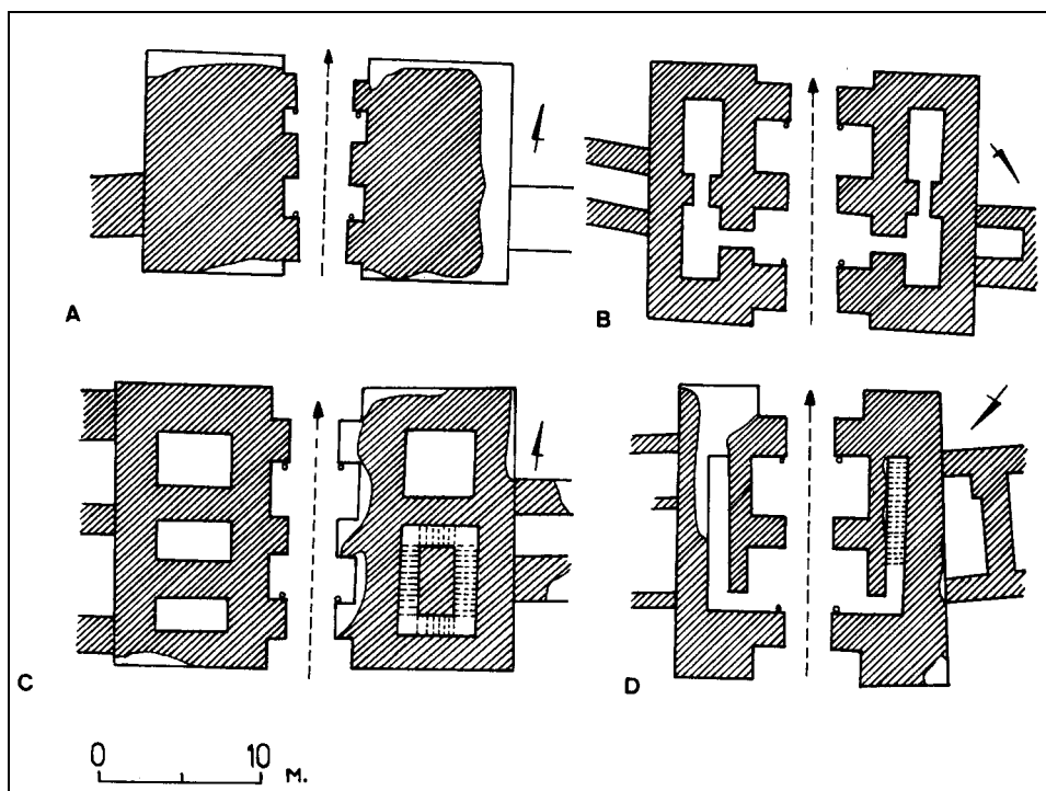
Klešťové brány střední doby bronzové IIB-C
