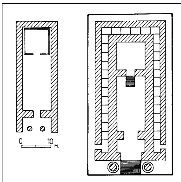
Šalomounův chrám v Jeruzalémě
