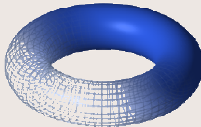
limitní torus
