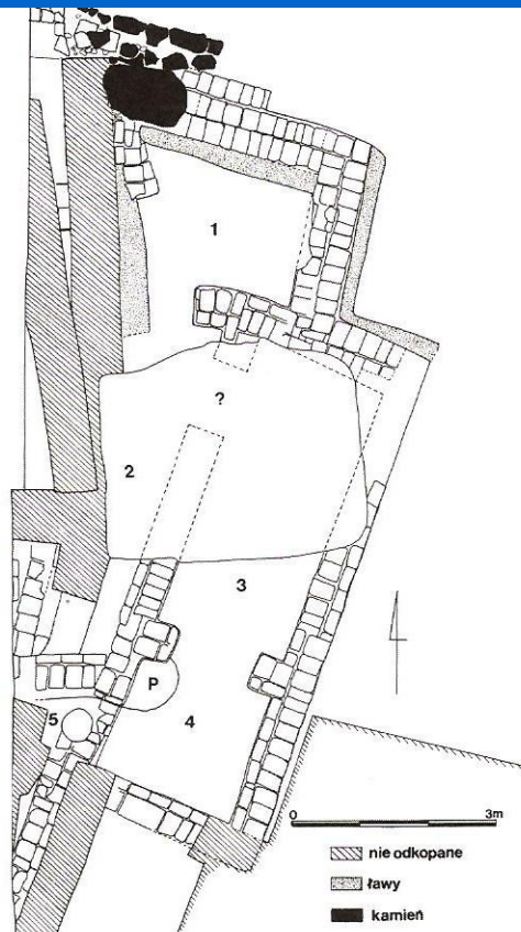
Ryc. 91. Tell Arbid, plan świątyni we wschodniej dzielnicy. Początek okresu wczesnodynastycznego III. Rys. M. Momot, D. Ławecka. P – palenisko.
