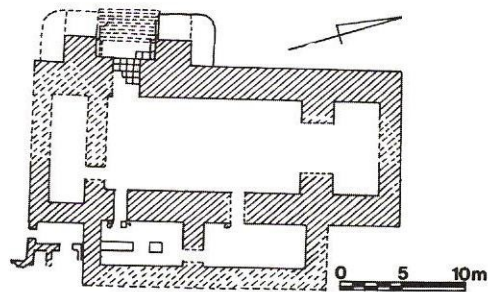
Ryc. 92. Aszur, plan świątyni Isztar (warstwa E, wg Andrae W. 1977, 112, fig. 89).
