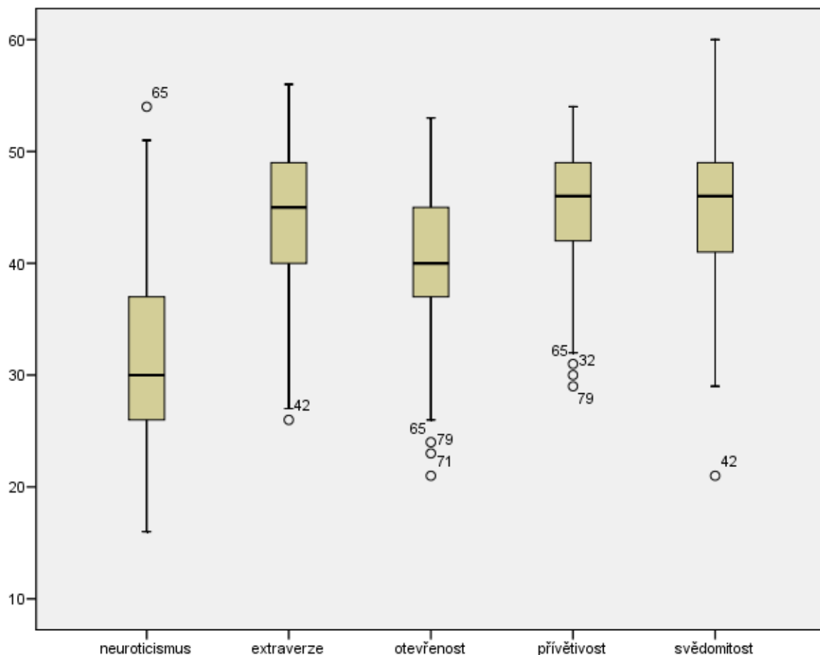
Graf 1. Rozdělení hodnot škál dotazníku NEO-FFI.
