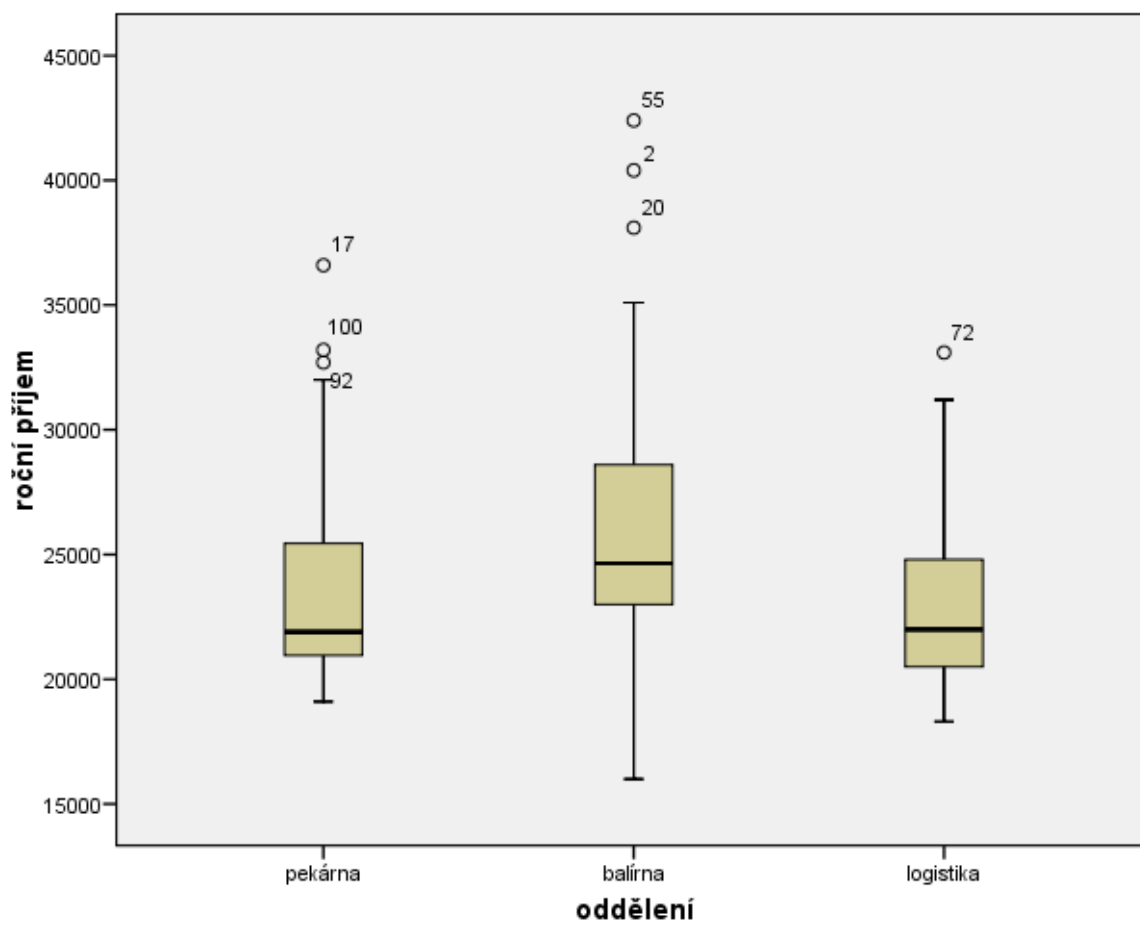
Graf 2. Porovnání hodnot ročního příjmu podle oddělení firmy.
