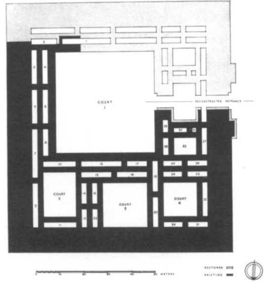
FIG. 2. Tell Braq. Plan of Naram-Sin Palace, ca. 2300 B.C. From Heinrich, Die Paläste , fig. 22.
